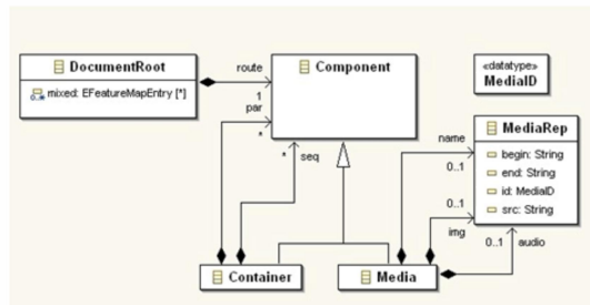
Pseudo language de classe (UML)
